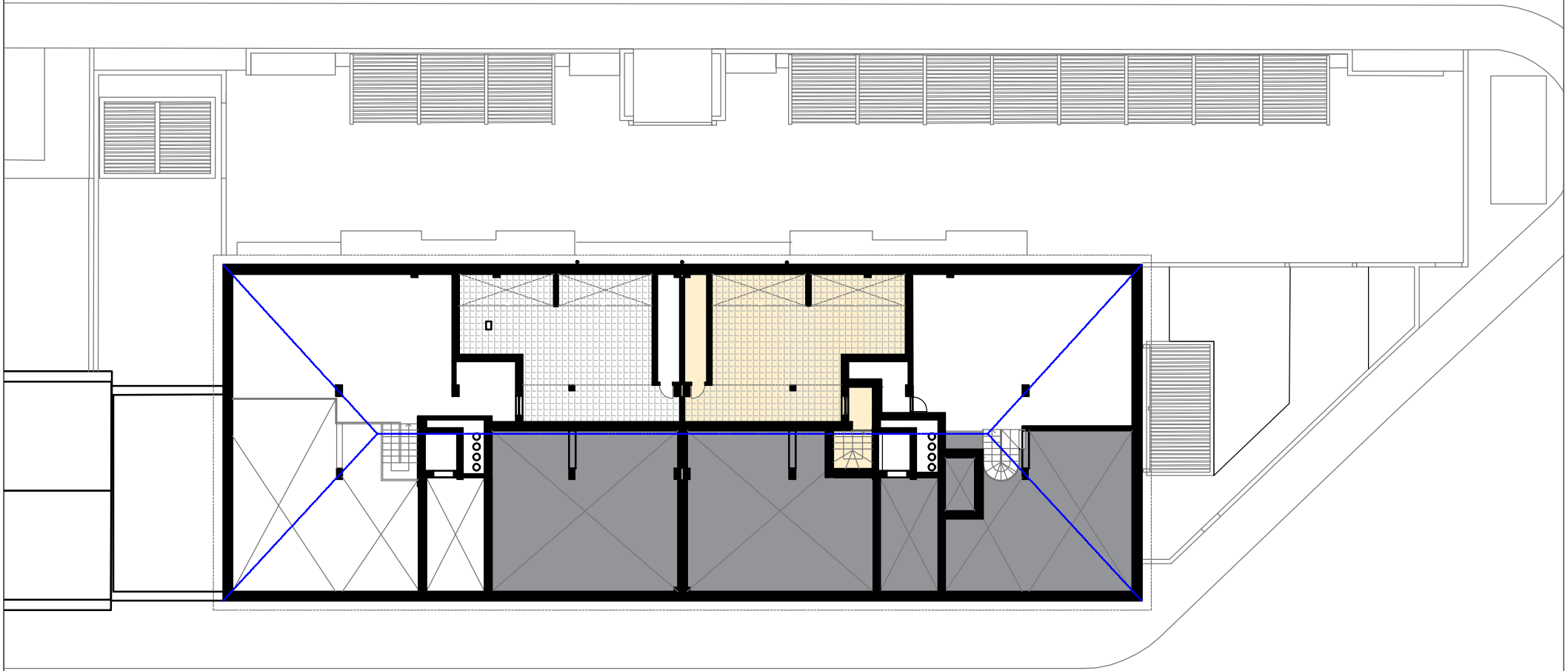
Planimetria piano sottotetto
