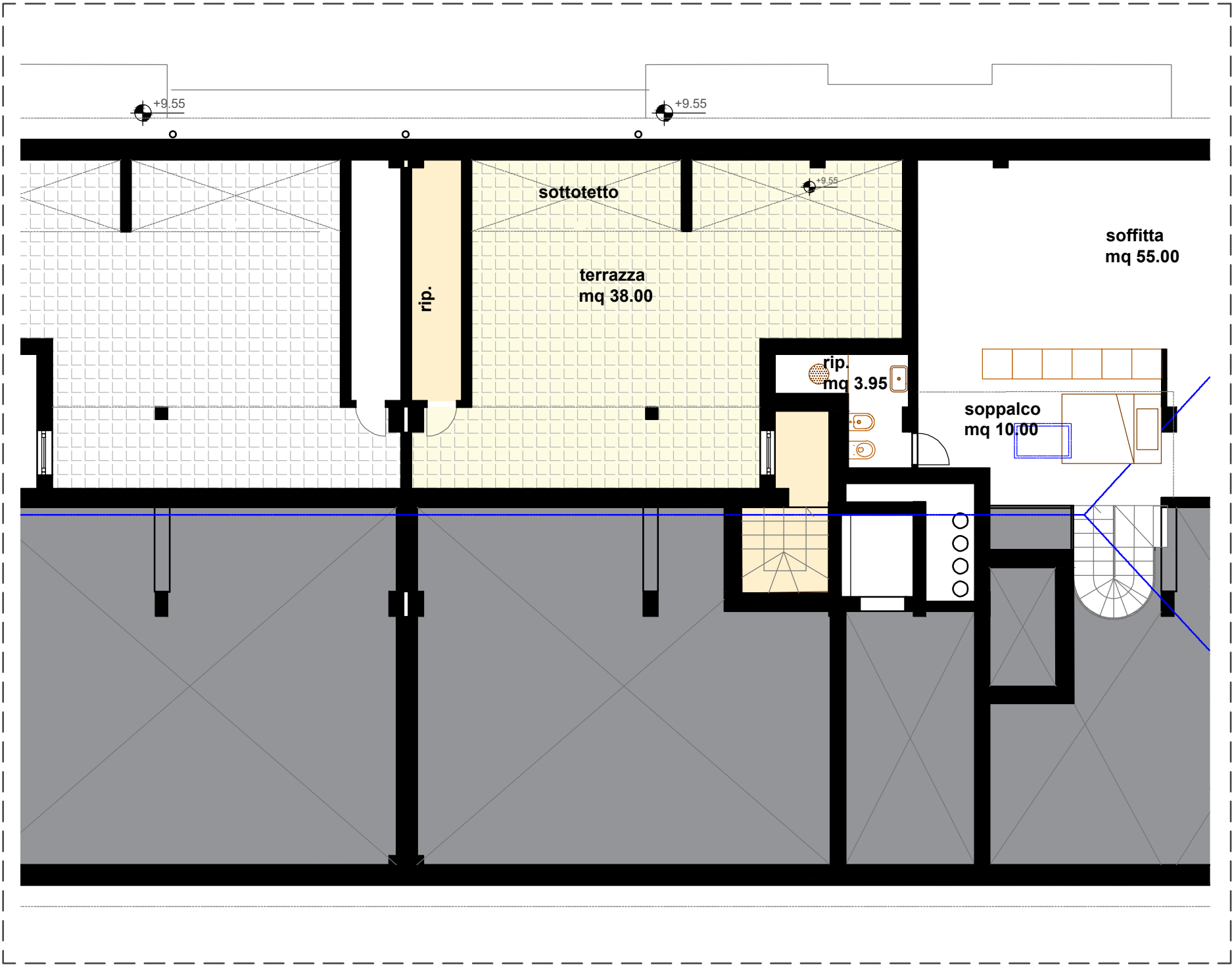
Planimetria piano sottotetto
